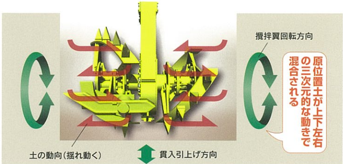
WILL工法(揺動攪拌)イメージ図
